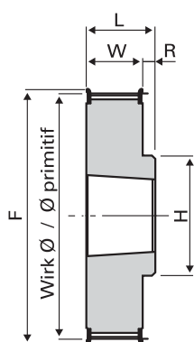
8RF Stahl/acier
